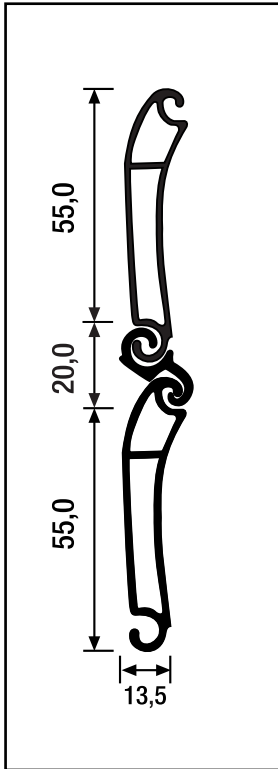
65 mm Lama aluminio extrusión doble pared. Perfil curvo autoblocante 65,0 mm
