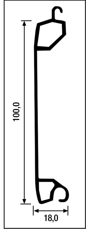
100 mm Lama aluminio extrusión monopared. Perfil curvo autoblocante 100,0 mm
