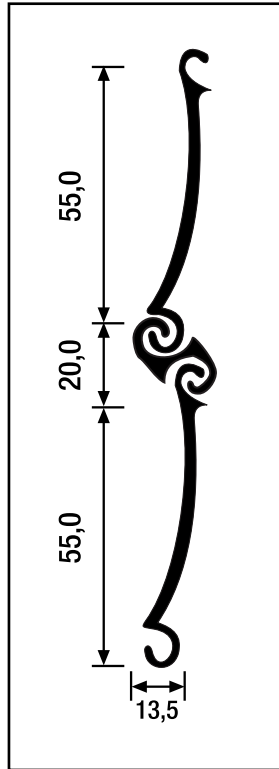
75 mm Lama aluminio extrusión monopared. Perfil curvo autoblocante 75,0 mm
