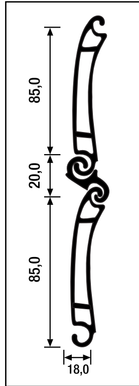
95 mm Lama aluminio extrusión doble pared. Perfil curvo autoblocante 95,0 mm
