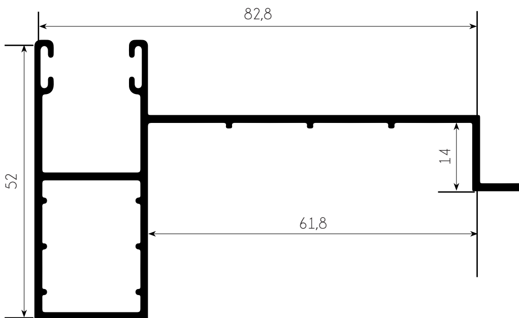
GUÍA R84-A
