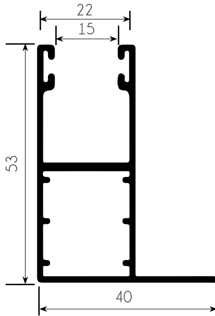
GUÍA H-40
