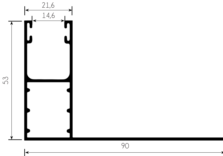
GUÍA H-90
