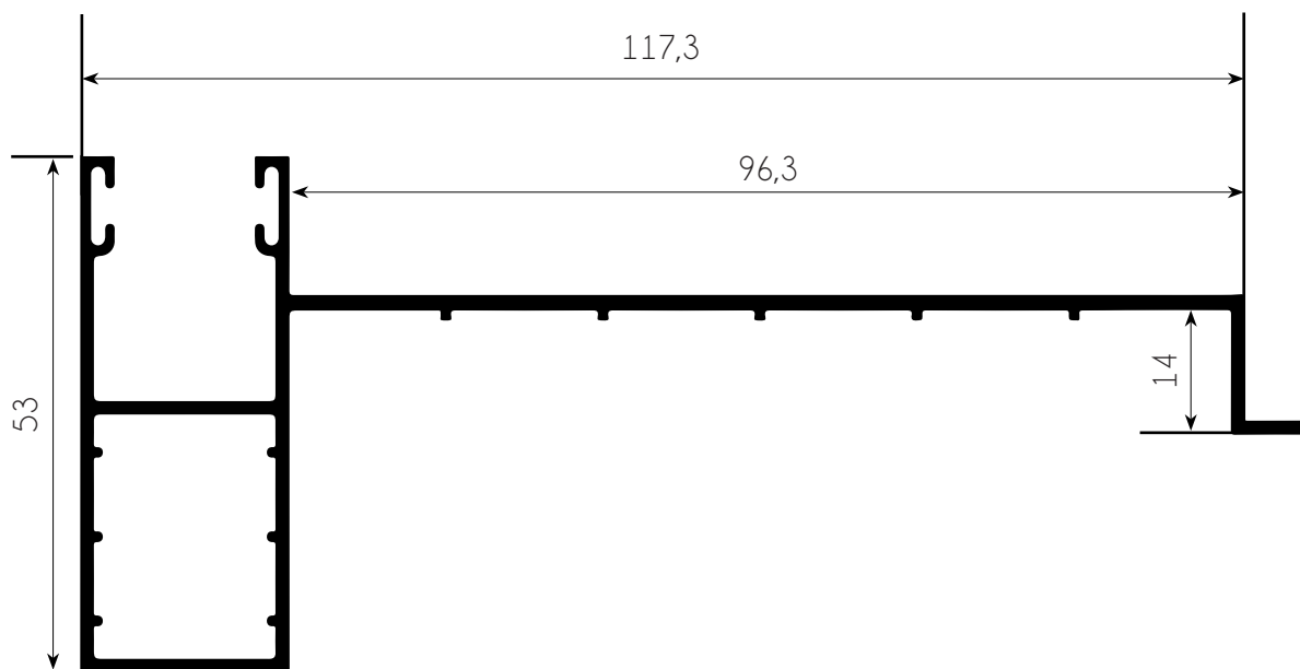
GUÍA R11-A
