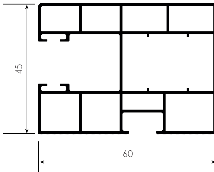
PVC 60X45
