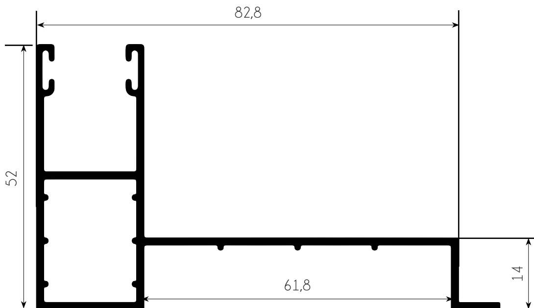
GUÍA R84-B
