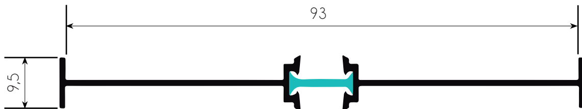
T-UNIÓN RPT-93
